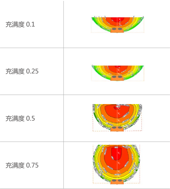
管径不同充满度的速度分布云图
