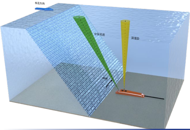
人工明渠流量监测
