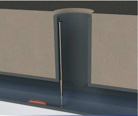
雨污水管网流量监测
